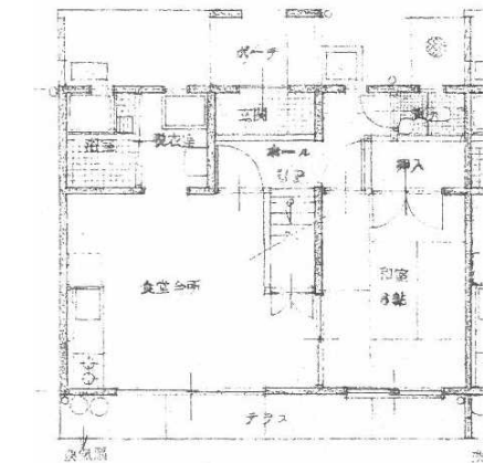
1階
