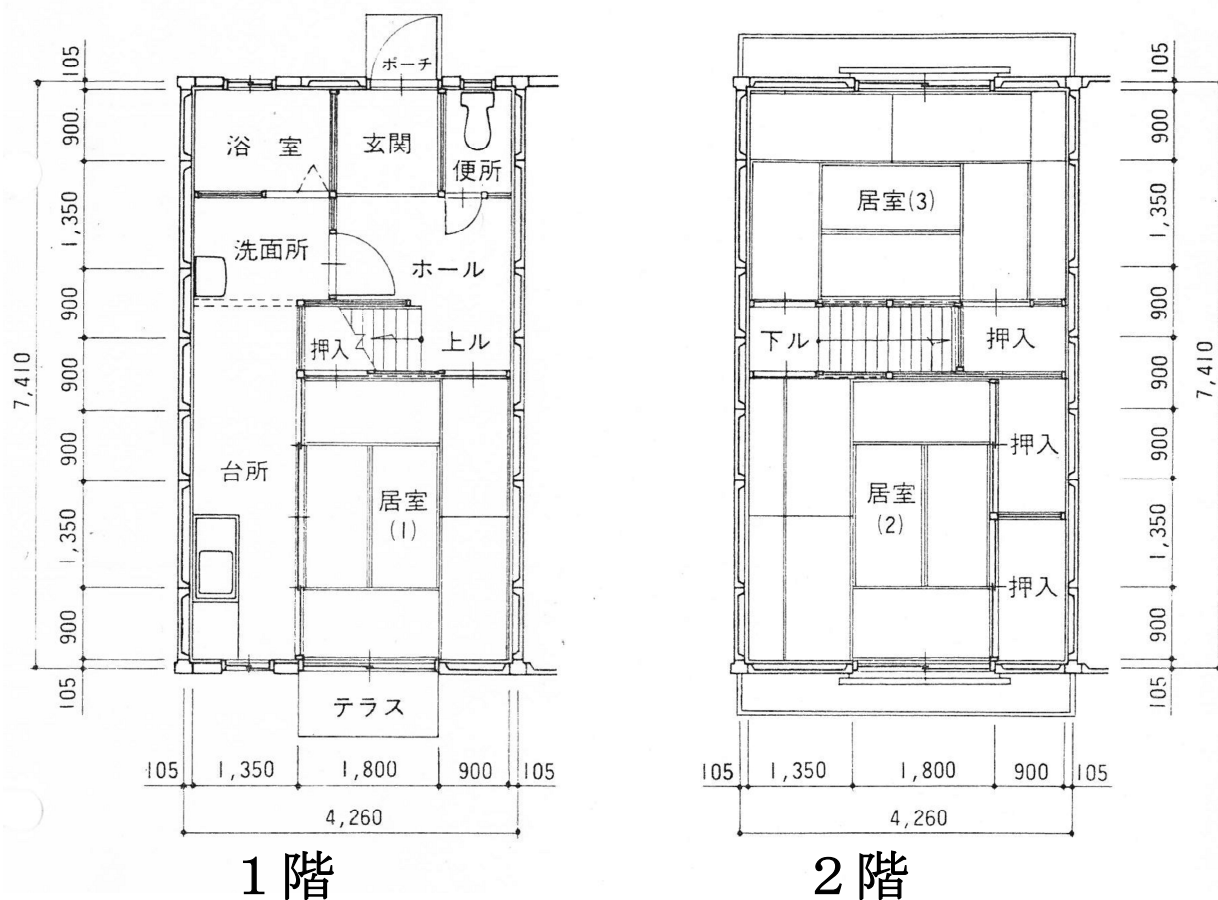
間取り図
