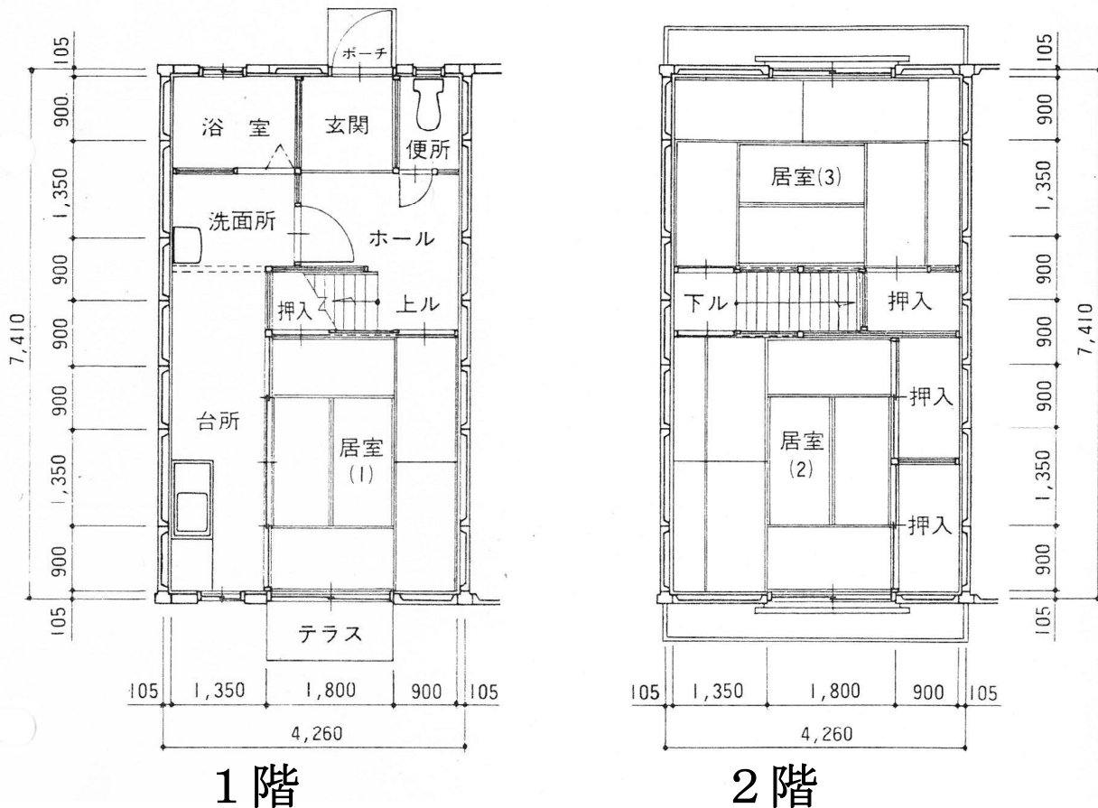
間取り図
